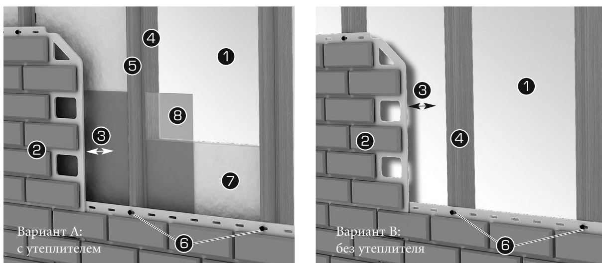
рис. 1: Варианты крепления обрешетки и фасадных панелей
