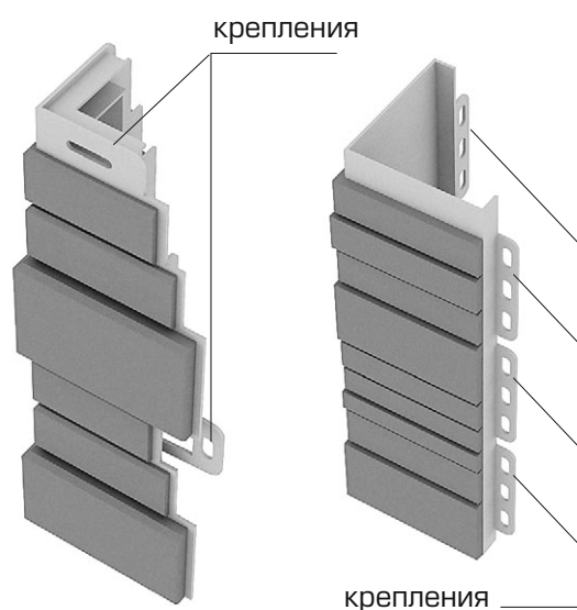
рис. 8: Наружный угол «Киpич Антик»
