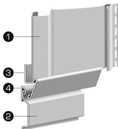
Рис. 6. Вариант стыковки вертикального и горизонтального сайдинга: 1 – вертикальный сайдинг; 2 – горизонтальный сайдинг; 3 – окантовочная планка; 4 – финишная планка.
